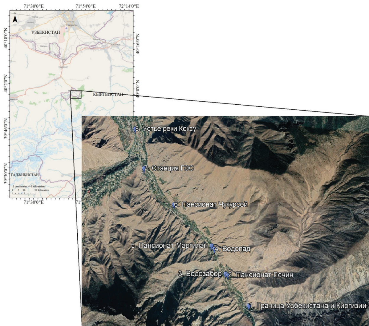
Рисунок 1 – Географическое расположение эксклава Шахимардан (слева) и космический снимок бассейна реки Коксу (высота н.у.м. – 1514 м – 1311 м) с указанием точек исследования ихтиофауны.
